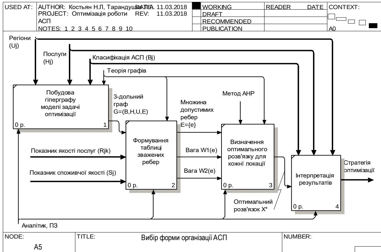
Рис. 3.7. Декомпозиція процесу «Вибір форми організації АСП»
