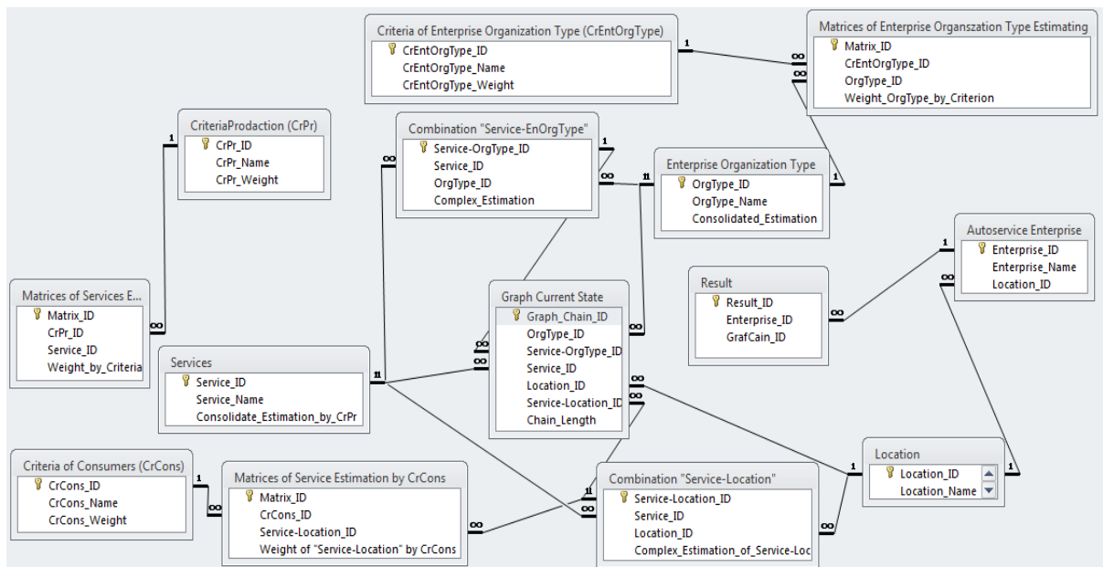
Рис. 4.14. Логічна модель бази даних підсистеми вибору оптимальної форми організації автосервісного підприємства
