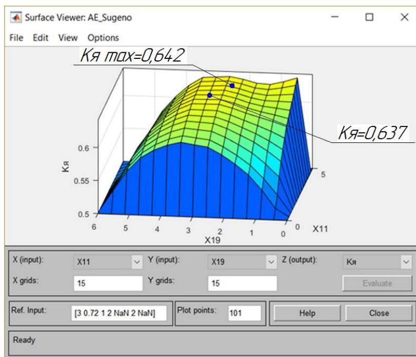
Рис. 5.55. Залежність K_{я} від типу енергетичних установок ( X_{11} ) та рівня доходу власників ТЗ ( X_{19} ) для авторизованого АСП
