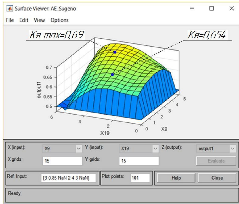
Рис. 5.38. Залежність K_y від форми організації виробництва ( X_9 ) та рівня доходу власників ТЗ ( X_{19} ) для пункту ТО
