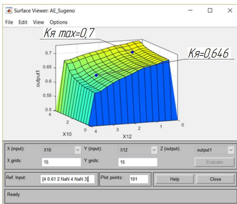
Рис. 5.30. Залежність коефіцієнта якості від повної маси автомобіля ( X_{10} ) та віку автомобілів ( X_{12} ) для спеціалізованого АСП
