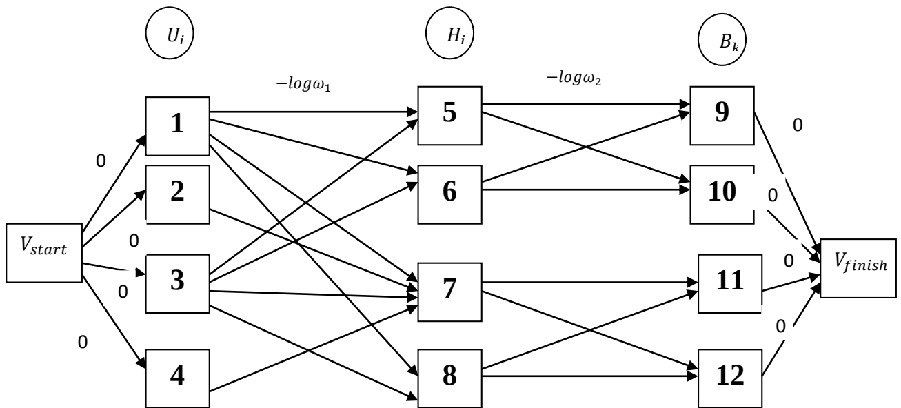
Рис. 4.13. Граф G' = (V', E')
