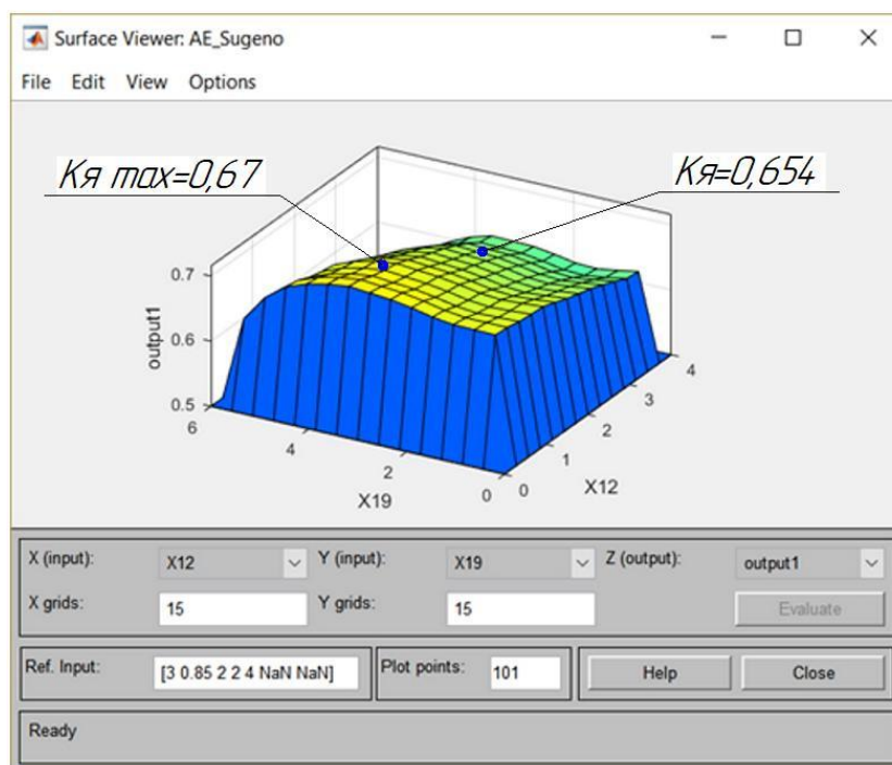
Рис. 5.41. Залежність K_{я} від віку автомобіля ( X_{12} ) та рівня доходу власників ТЗ ( X_{19} ) для пункту ТО
