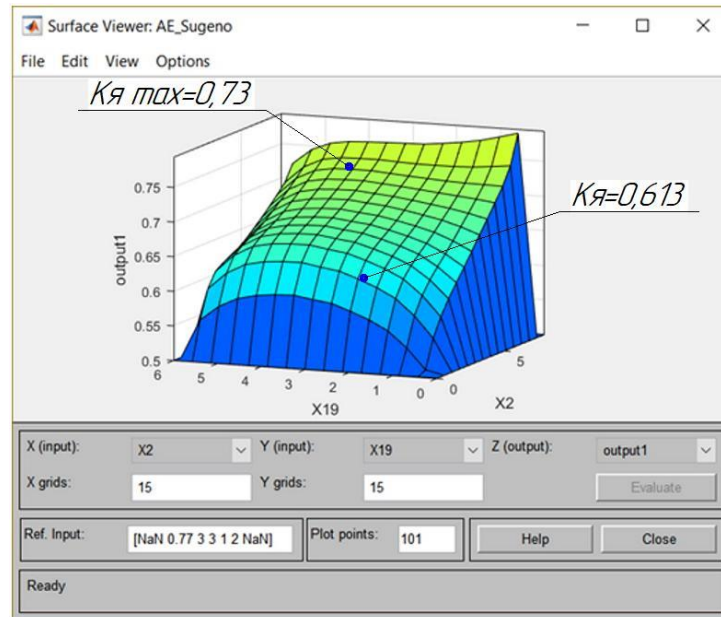
Рис. 5.43. Залежність K_{я} від потужності АСП ( X_2 ) та рівня доходу власників ТЗ ( X_{19} ) для авторемонтної майстерні
