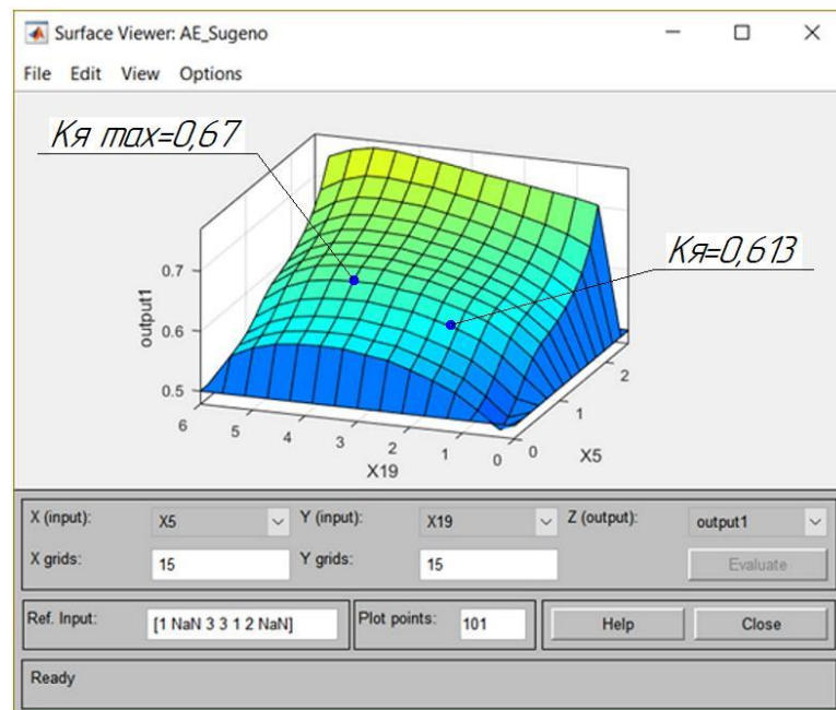
Рис. 5.44. Залежність K_{я} від рівня забезпеченості персоналом ( X_5 ) та рівня доходу власників ТЗ ( X_{19} ) для авторемонтної майстерні
