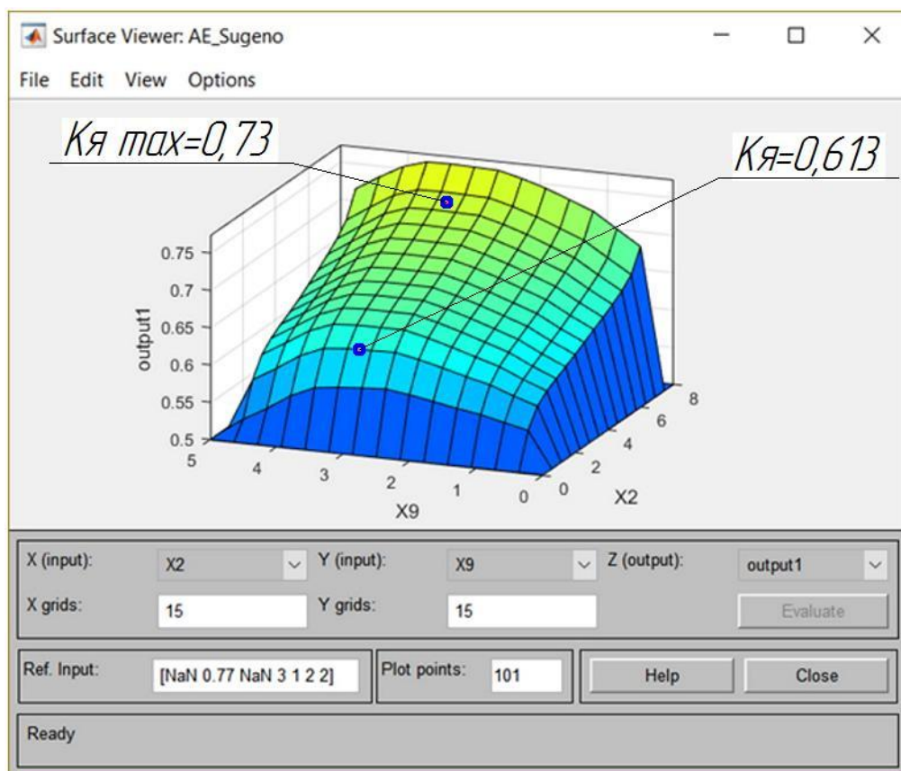
Рис. 5.7. Залежність коефіцієнта якості від потужності АСП ( X_2 ) та форми організації виробництва ( X_9 ) для авторемонтних майстерень
