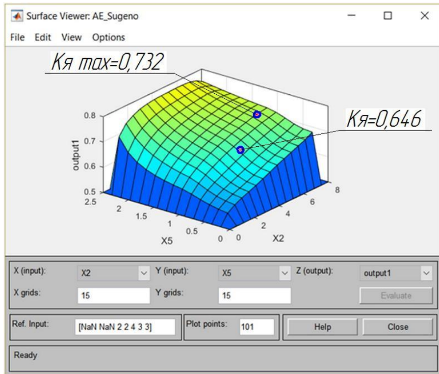
Рис. 5.18. Залежність коефіцієнту якості від потужності АСП ( X_2 ) та рівня забезпеченості персоналом ( X_5 ) для спеціалізованого АСП
