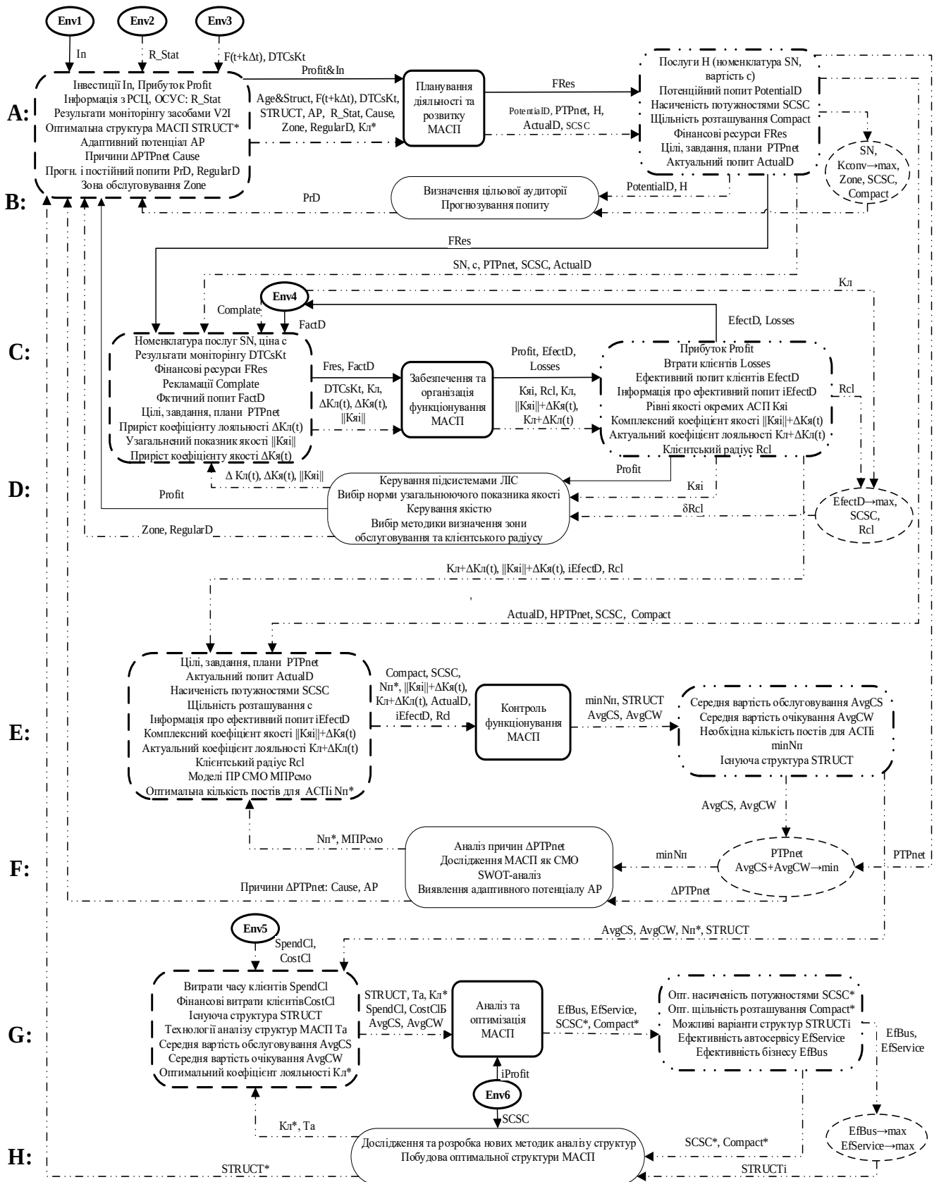
Рис. 2.5. Структура моделі системи автосервісу на метарівні
