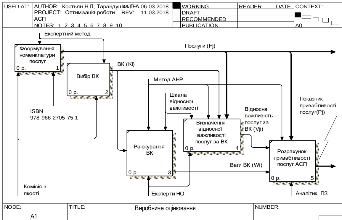
Рис. 3.4. Декомпозиція процесу «Виробниче оцінювання»
