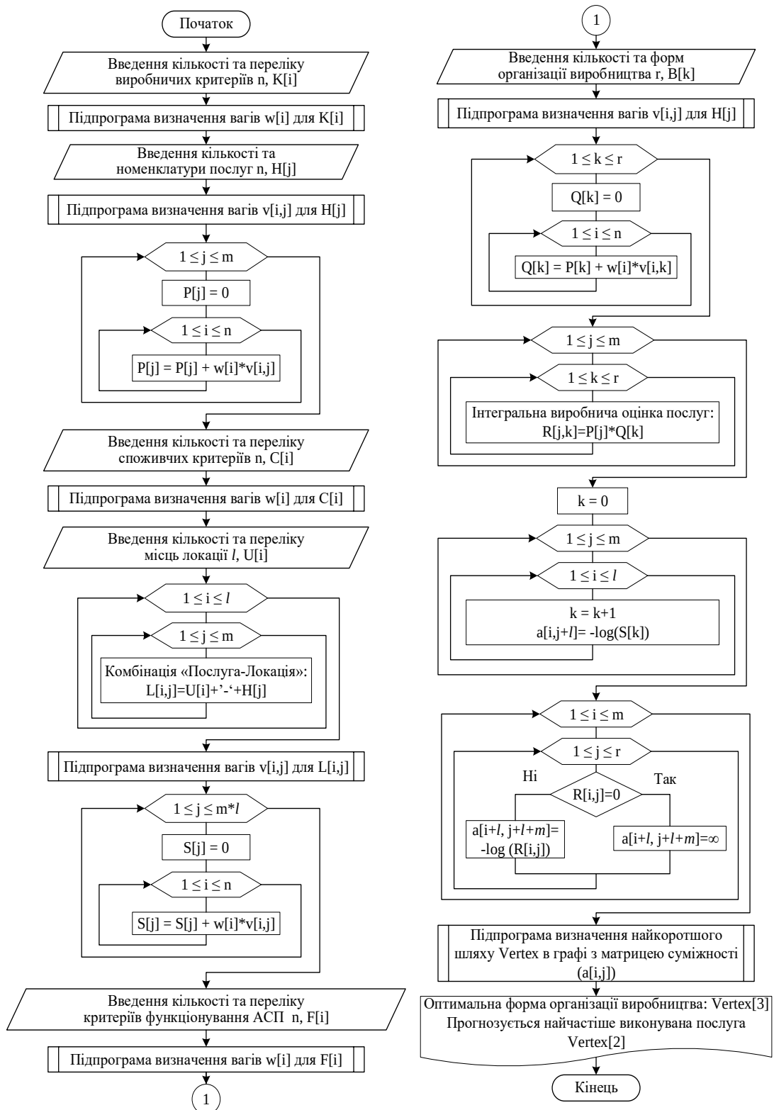
Рис. 3.8. Блок-схема алгоритму визначення оптимальної форми організації
