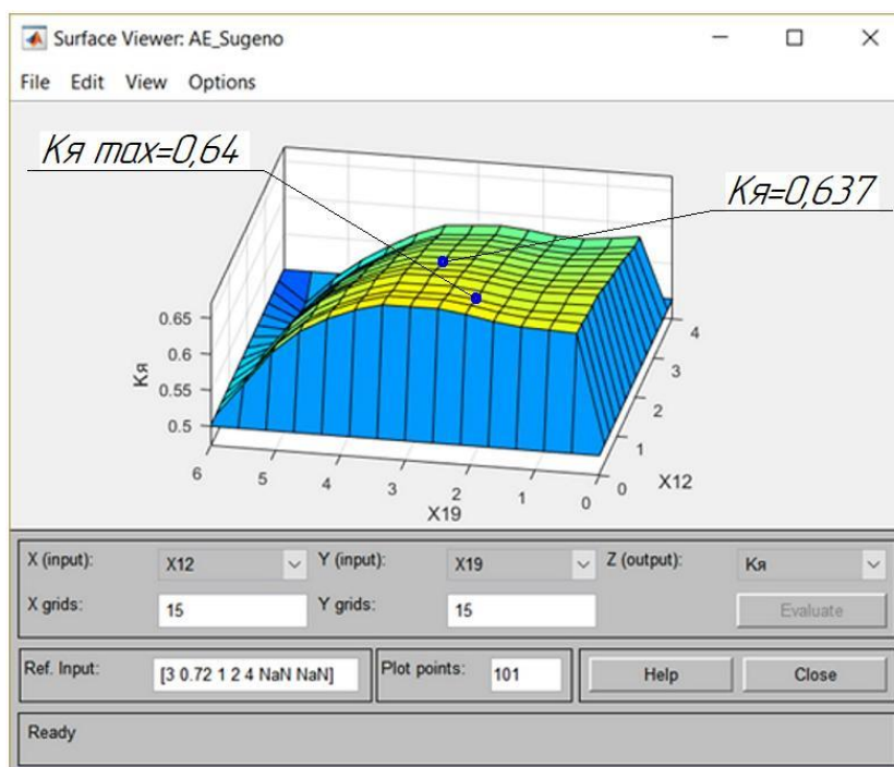
Рис. 5.56. Залежність K_{я} від віку автомобіля ( X_{12} ) та рівня доходу власників ТЗ ( X_{19} ) для авторизованого АСП
