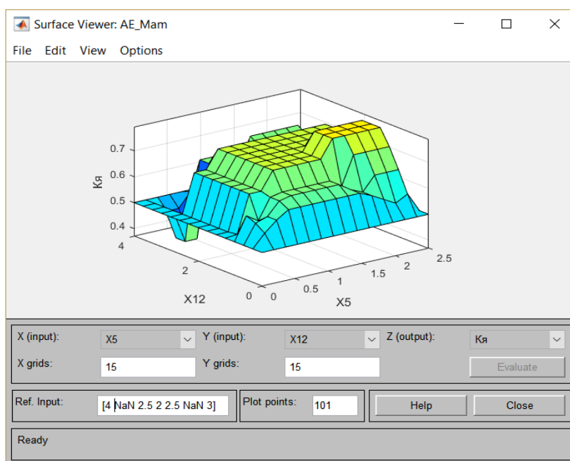
Рис. 4.9. Залежність K_{\text{я}} від рівня забезпеченості персоналом та середнього віку автомобілів в системі типу Мамдані
