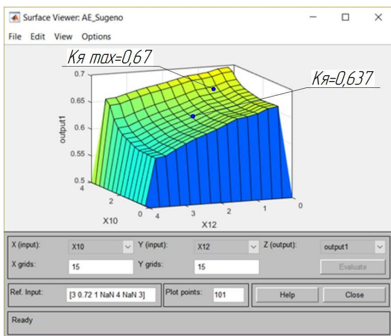
Рис. 5.29. Залежність коефіцієнта якості від повної маси автомобіля ( X_{10} ) та віку автомобілів ( X_{12} ) авторизованого СТО
