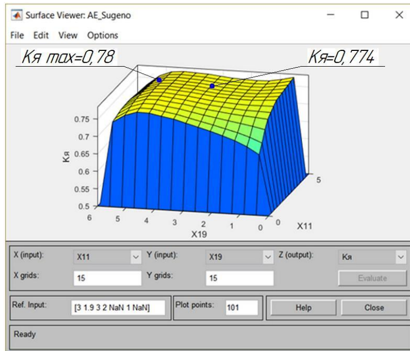
Рис. 5.64. Залежність K_{я} від типу енергетичних установок ( X_{11} ) та рівня доходу власників ТЗ ( X_{19} ) для комплексного АСП
