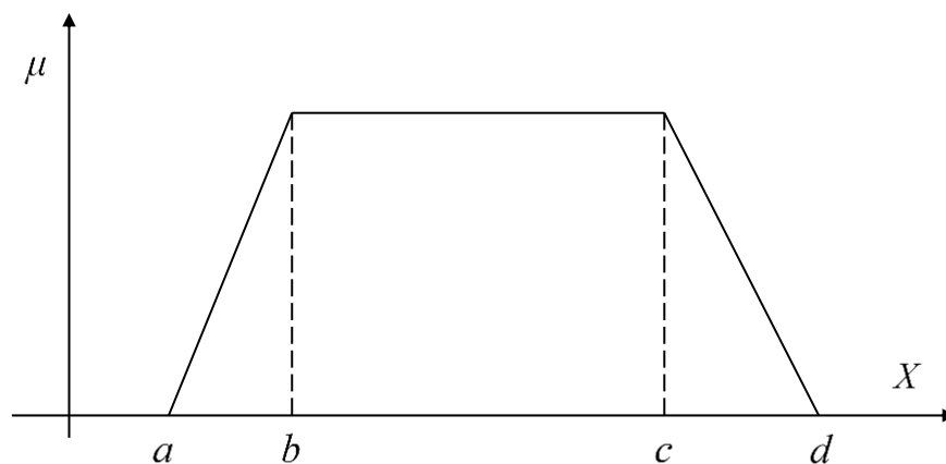
Рис. 4.3. Загальний вигляд трапецієподібної функції належності
