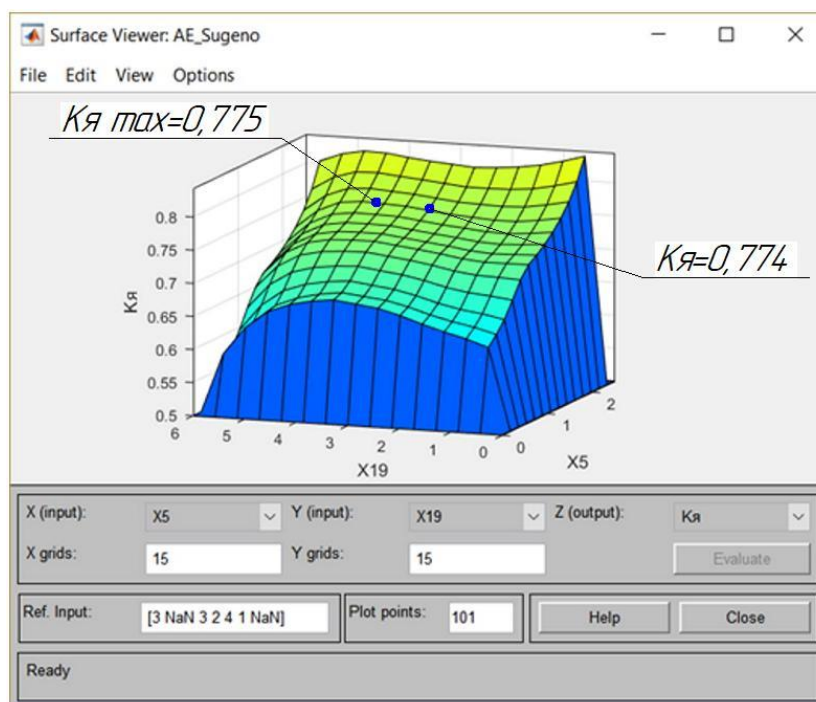
Рис. 5.62. Залежність K_{я} від рівня забезпеченості персоналом ( X_5 ) та рівня доходу власників ТЗ ( X_{19} ) для комплексного АСП
