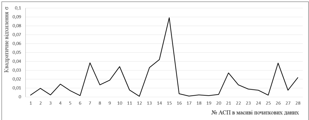
Рис. 4.2. Похибка лінійної моделі, що побудовано на початковій виборці
