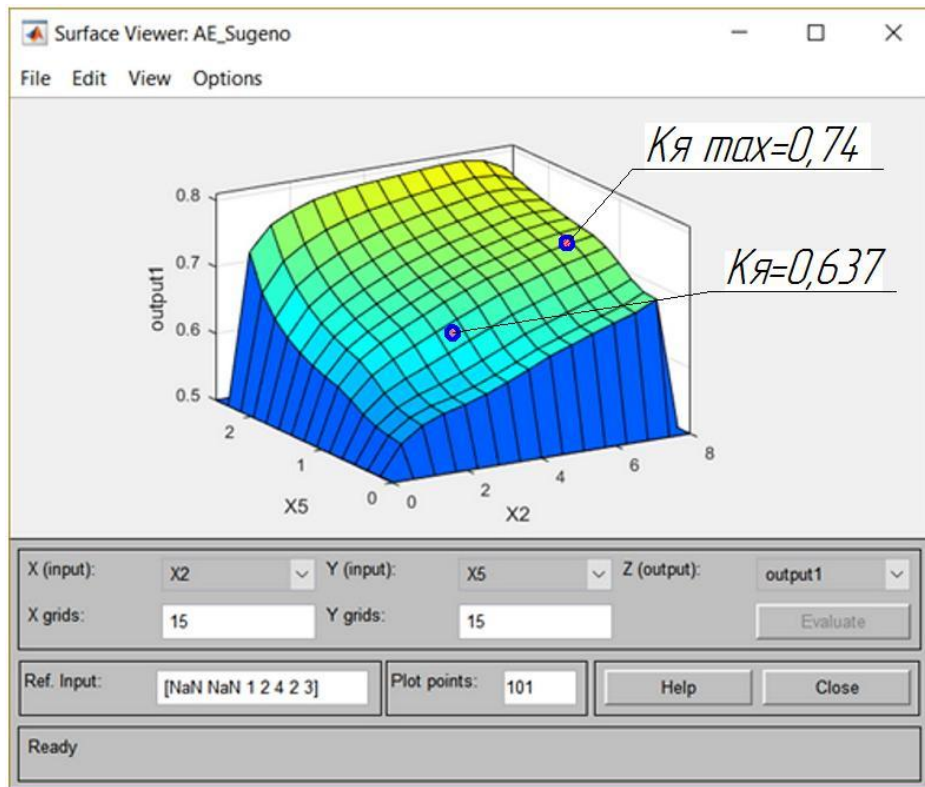
Рис. 5.14. Залежність коефіцієнту якості від потужності АСП ( X_2 ) та рівня забезпеченості персоналом ( X_5 ) для авторизованої СТО
