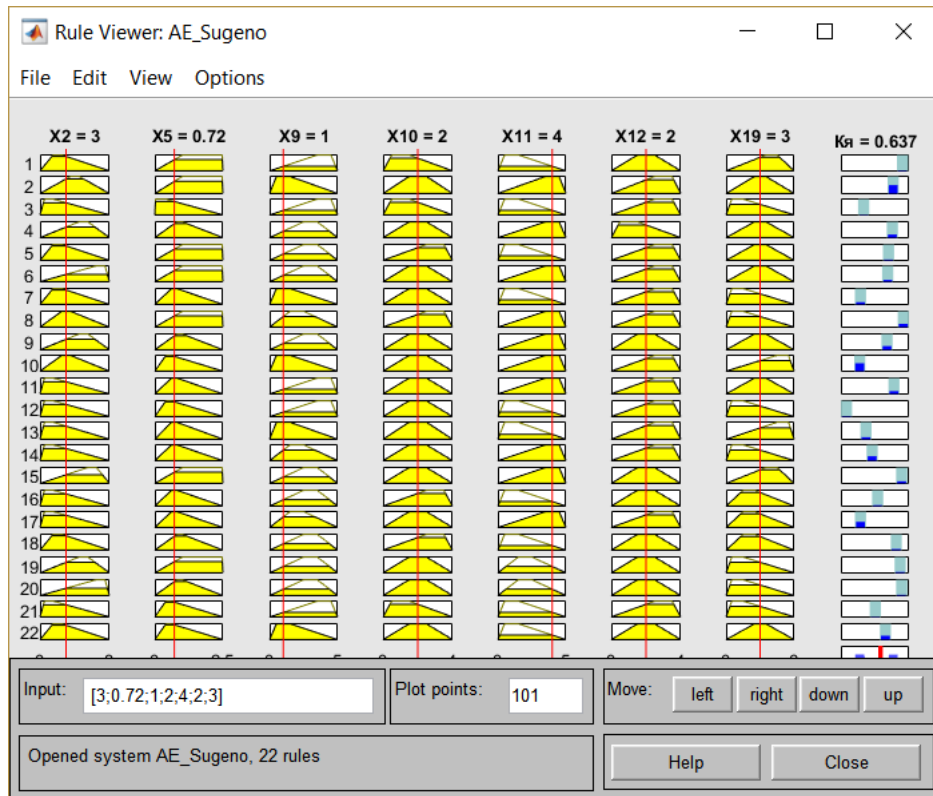
Рис. 5.13. Візуалізація логічного виведення K_{\text{я}} авторизованого СТО ТОВ «Дніпромотор», м. Дніпро
