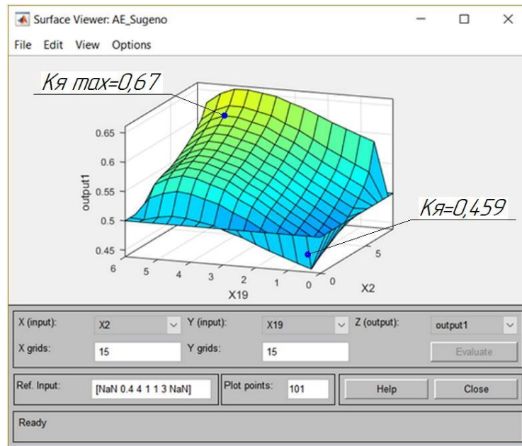
Рис. 5.45. Залежність коефіцієнта якості від потужності АСП ( X_2 ) та рівня доходу власників ТЗ ( X_{19} ) для СТО
